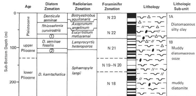
① Actinocyclus oculatus ② Denticula seminiae fossilis — D. kamtschatica
